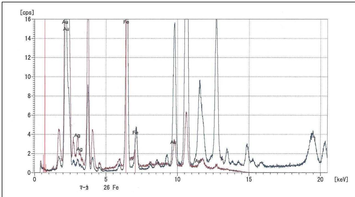
図 3 : 同 寛政期金箔の蛍光 X 線分析結果
