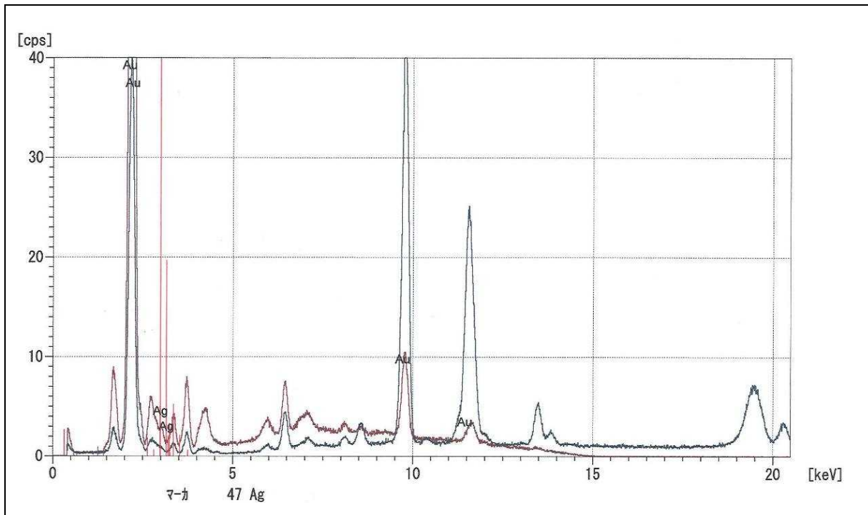
図 1 : 同 寛永期金箔の蛍光 X 線分析結果
