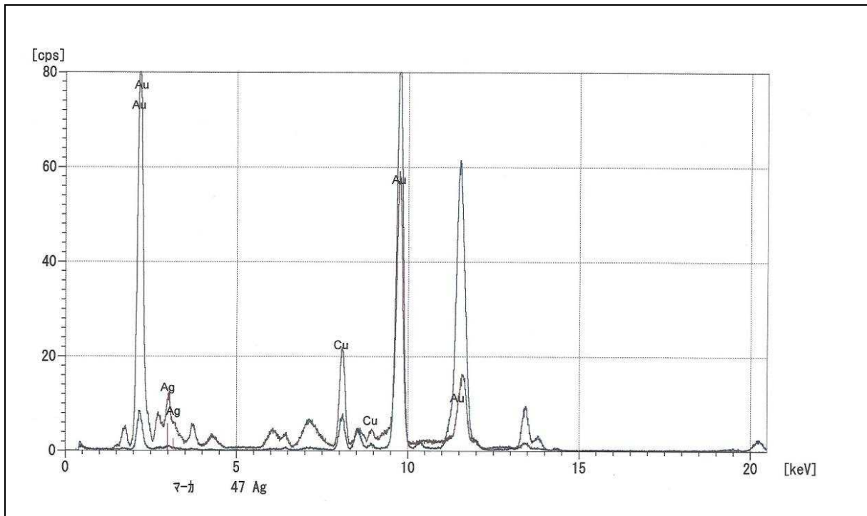
図 4 : 甲州一分金の蛍光 X 線分析結果
