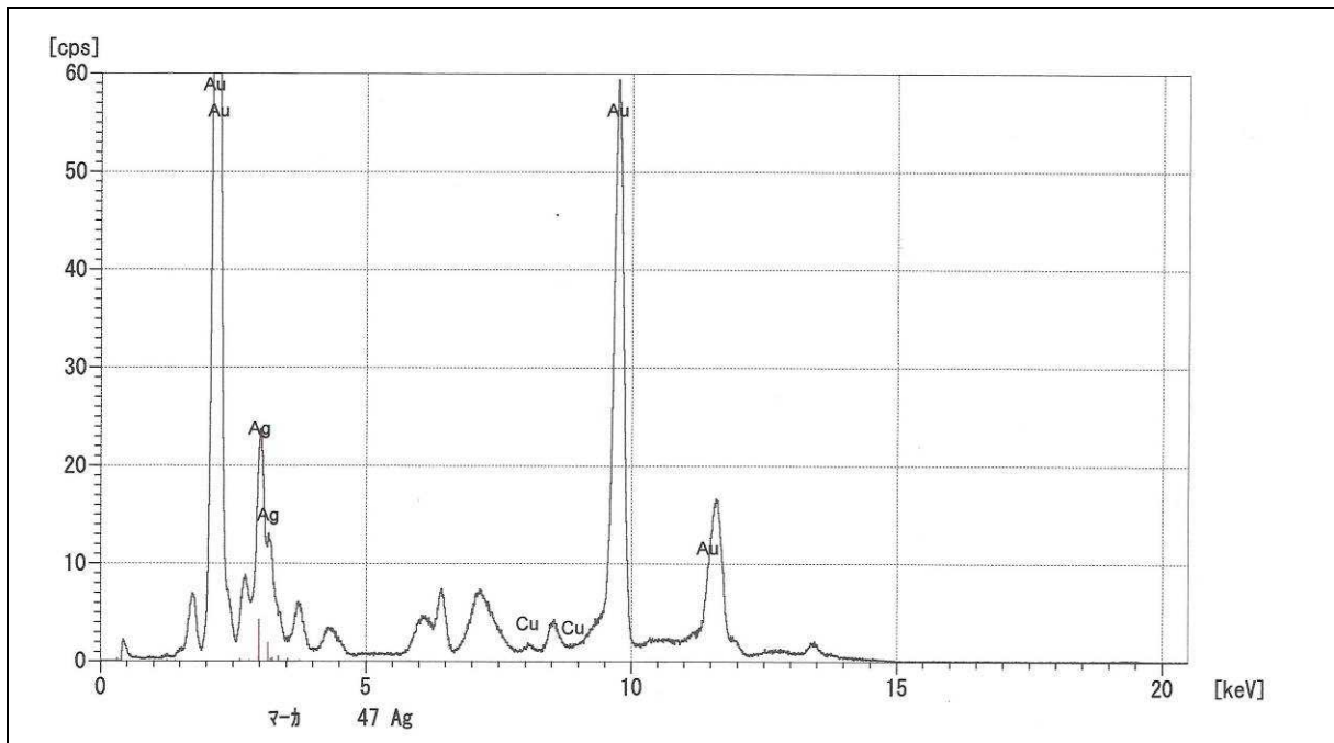
図 5 : 元禄一分金の蛍光 X 線分析結果
