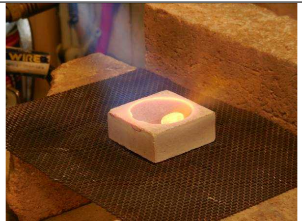
写真 13 : インゴットの作成②
