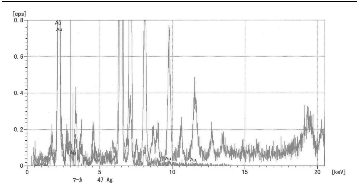
図 2 : 同 寛政期金箔の蛍光 X 線分析結果
