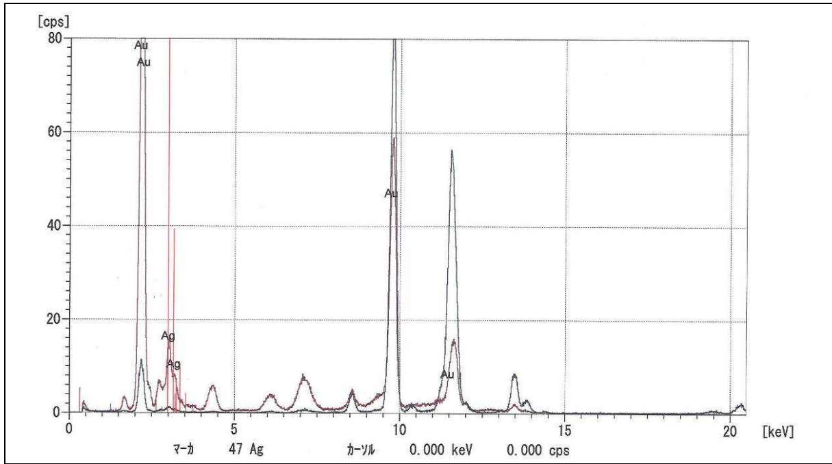
図 6 : 復元焦箔の蛍光 X 線分析結果
